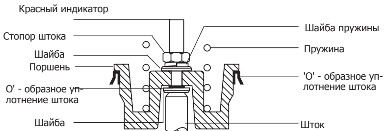
Рис. 6 Нормально закрытый клапан (NC)
