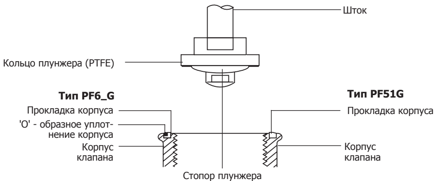
Рис. 9 Поставляемые запчасти
