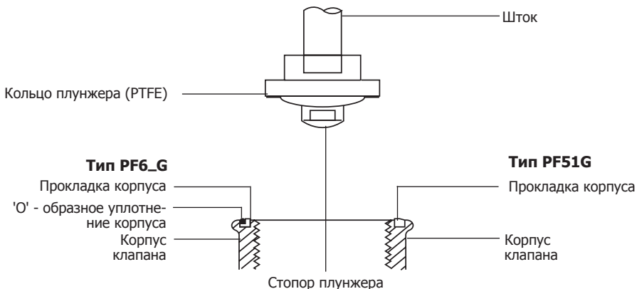
Рис. 8 Клапан двойного действия (BD)
