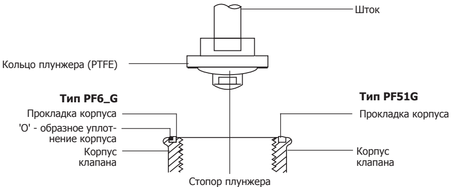
Рис. 9 Поставляемые запчасти
